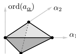
ABBILDUNG 2. Erweitertes NP
