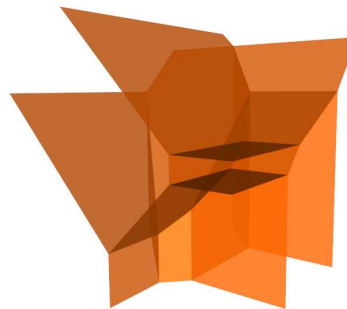
ABBILDUNG 5. tropische Quadrik
