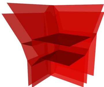
ABBILDUNG 6. tropische Kubik
