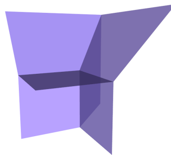
ABBILDUNG 4. tropische Ebene
