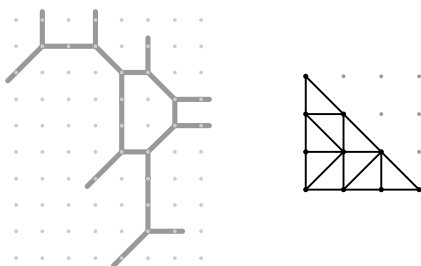
ABBILDUNG 3. tropische Kubik
