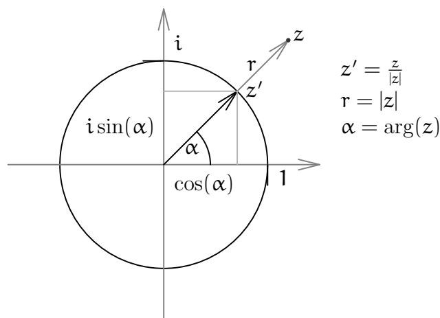
ABBILDUNG 4. Polarkoordinaten von z = r \cdot (\cos(\alpha) + i \cdot \sin(\alpha))
