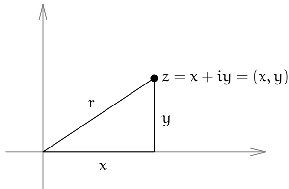
ABBILDUNG 2. Pythagoras: x^2 + y^2 = r^2
