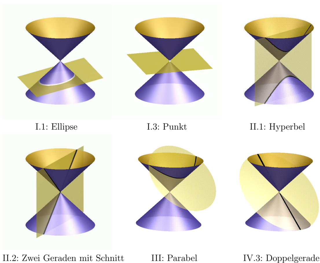
ABBILDUNG 1. Kegelschnitte
