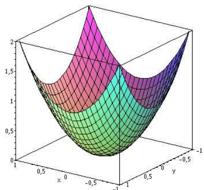
f''(0,0) positiv definit lokales Minimum
