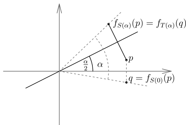
ABBILDUNG 11. Die Spiegelung S(\alpha) = T(\alpha) \circ S(0)
