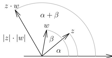
ABBILDUNG 7. Multiplikation zweier komplexer Zahlen
