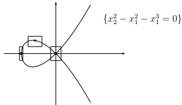
ABBILDUNG 9. Die Lösungsmenge von x_2^2 - x_1^2 - x_1^3 = 0
