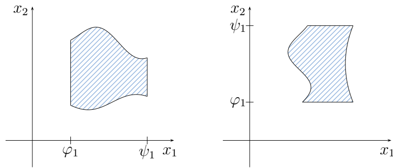
ABBILDUNG 25. Normalbereiche bez. (x_1, x_2) und bez. (x_2, x_1)
