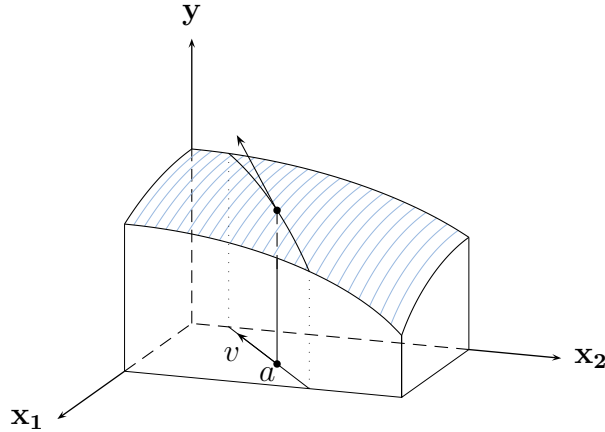
ABBILDUNG 4. Richtungsableitung \frac{\partial f}{\partial v}(a) in Richtung v
