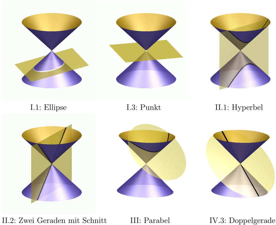
ABBILDUNG 16. Kegelschnitte
