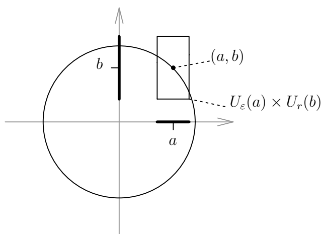
ABBILDUNG 10. Die Kreislinie \{x^2 + y^2 - 1 = 0\}
