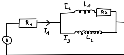
ABBILDUNG 13. Gekoppelter elektrischer Schwingkreis
