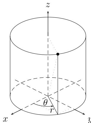
ABBILDUNG 32. Zylinderkoordinaten
