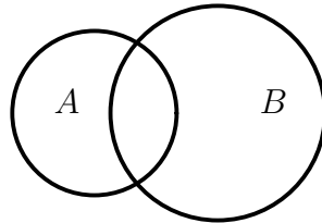
ABBILDUNG 24. \partial(A \cup B), \partial(A \cap B), \partial(A \setminus B) \subseteq \partial A \cup \partial B
