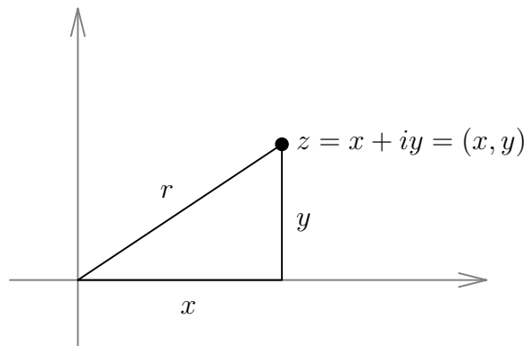
ABBILDUNG 4. Pythagoras: x^2 + y^2 = r^2
