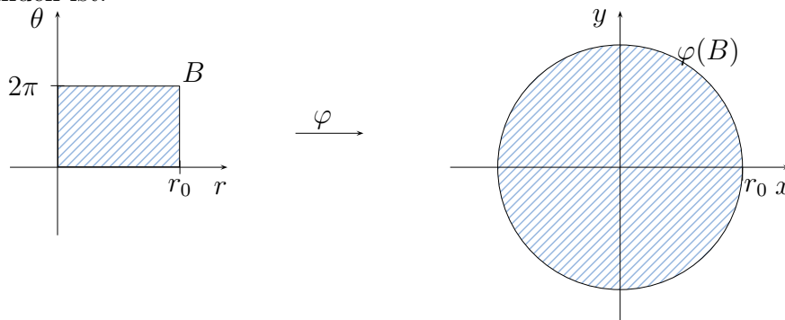
ABBILDUNG 30. Transformation eines Rechtecks auf einen Kreis
