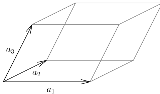
ABBILDUNG 28. Das Parallelotop P(a_1, a_2, a_3) im \mathbb{R}^3
