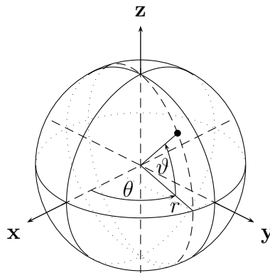
ABBILDUNG 33. Kugelkoordinaten
