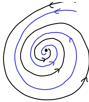
ABBILDUNG 18. Linearer Fluß zu \sigma(A) = \{\alpha \pm i\beta\} mit \alpha < 0 < \beta
