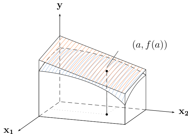
ABBILDUNG 5. Tangentialraum an den Graphen von f in (a, f(a))
