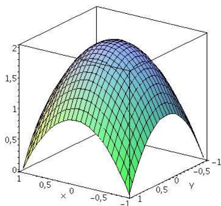
anschaulich: Volumen zwischen z = f(x, y) und xy -Ebene
